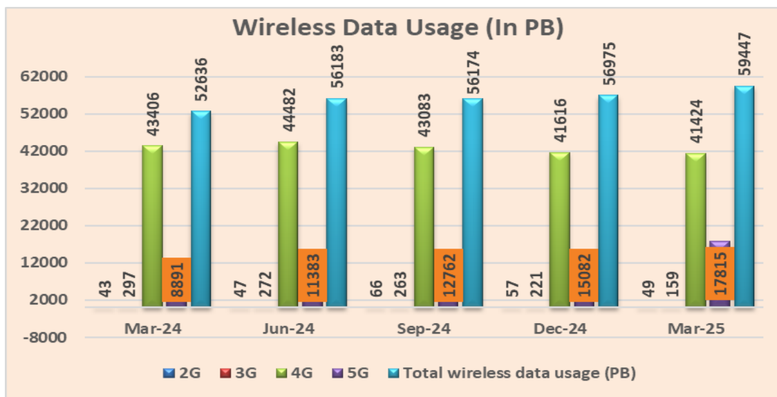
चार्ट 1.10: प्रौद्योगिकी के लिहाज से वायरलेस डेटा उपयोग का रुझान (पीबी में)
